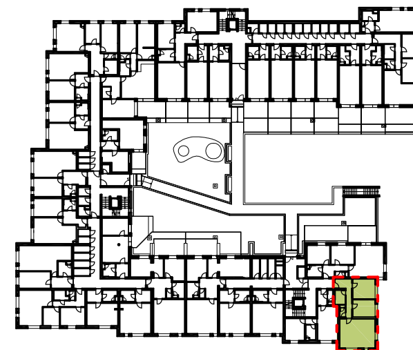
Schéma podlaží
